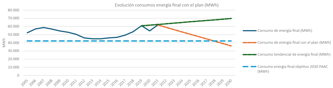
Figura 62. Evolución de los consumos de energía final esperadas en El Saucejo con la aplicación del PMCC. Fuente: Elaboración propia
