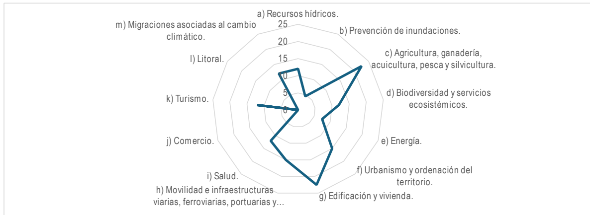
Figura 47. Diagrama resumen de las valoraciones del riesgo del impacto "cambios en la frecuencia, intensidad y magnitud de los incendios forestales" en las áreas estratégicas seleccionadas en El Saucejo.
