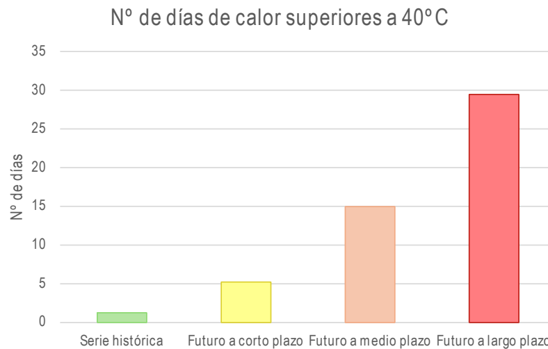
Figura 39. Diagrama de variación del número de días en los que se superan los 40 °C al año en El Saucejo para la serie histórica de 1961 a 1990 y para los horizontes temporales de futuro a corto, medio y largo plazo.
