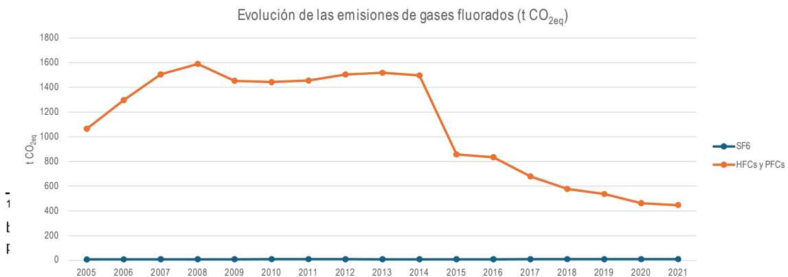
Figura 17. Evolución de las emisiones de los gases fluorados por tipo de 2005 a 2021.
